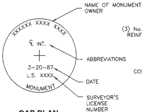
CAP PLAN
