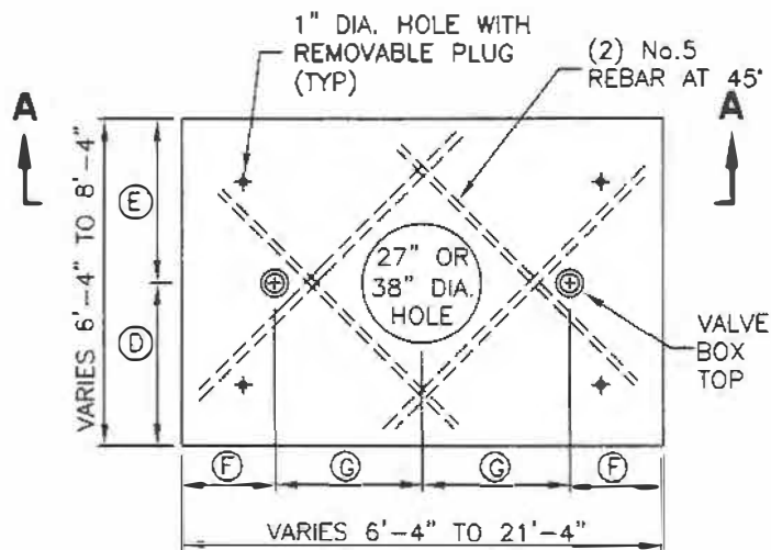
LID PLAN
