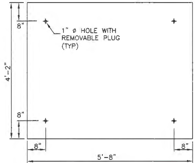
LID PLAN
