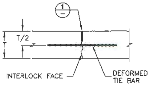
T-1 INTERLOCK FACE
