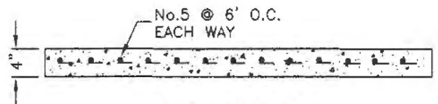
LID SECTION
